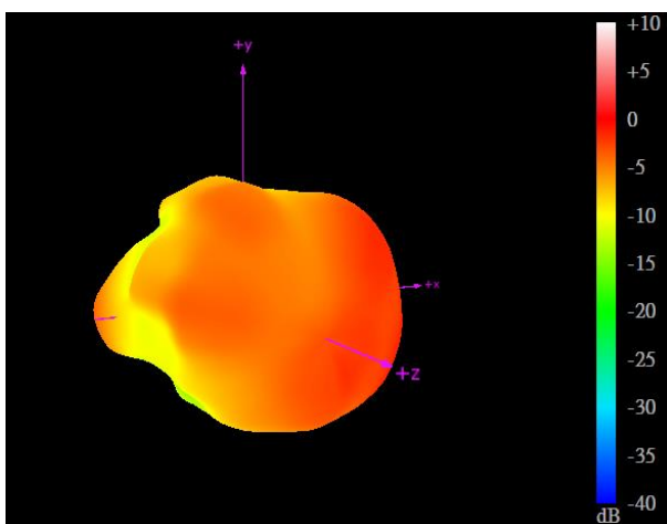
1710MHz
