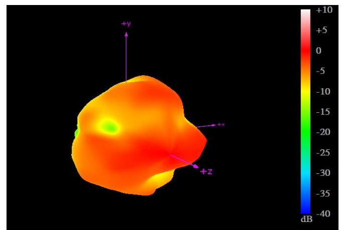
3500MHz
