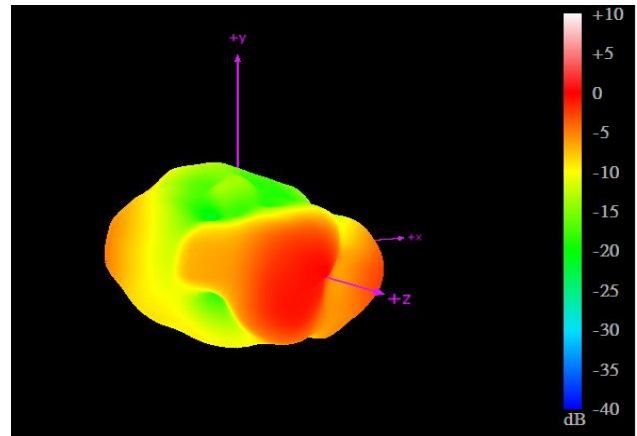
2170MHz
