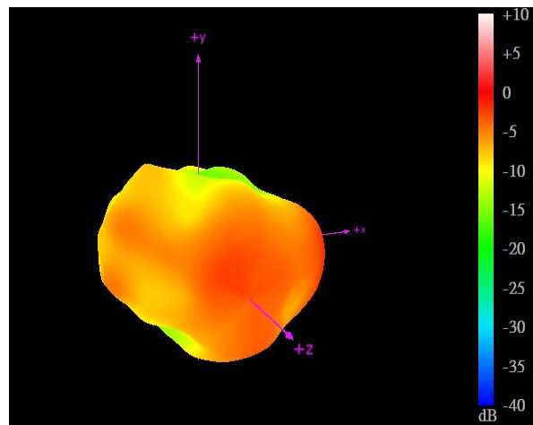
2170MHz
