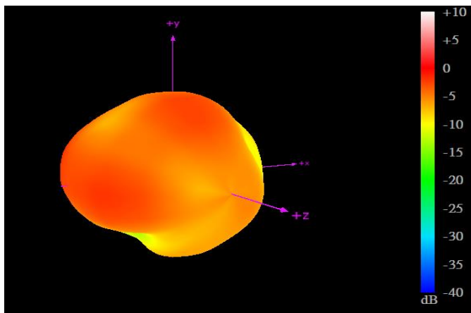
704MHz
