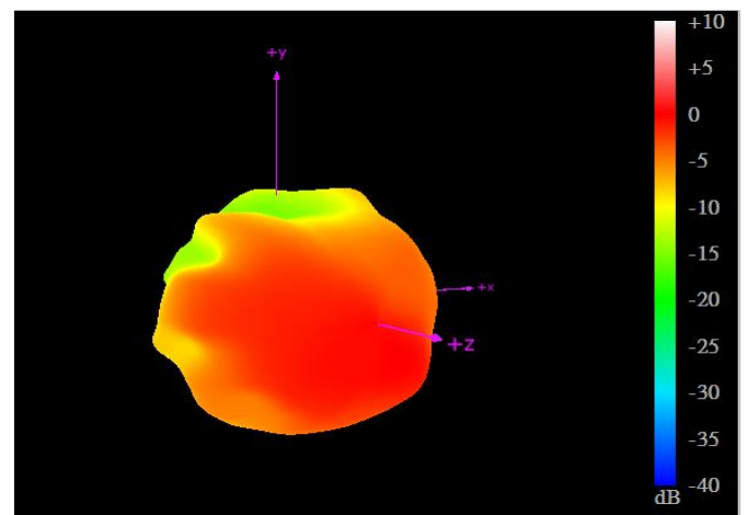
2170MHz
