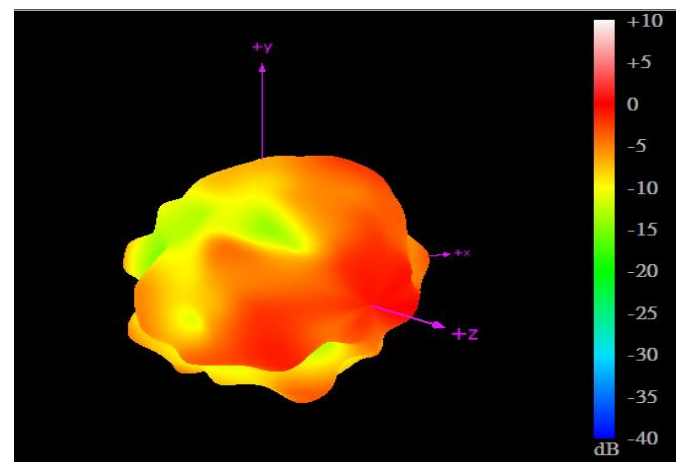
3500MHz
