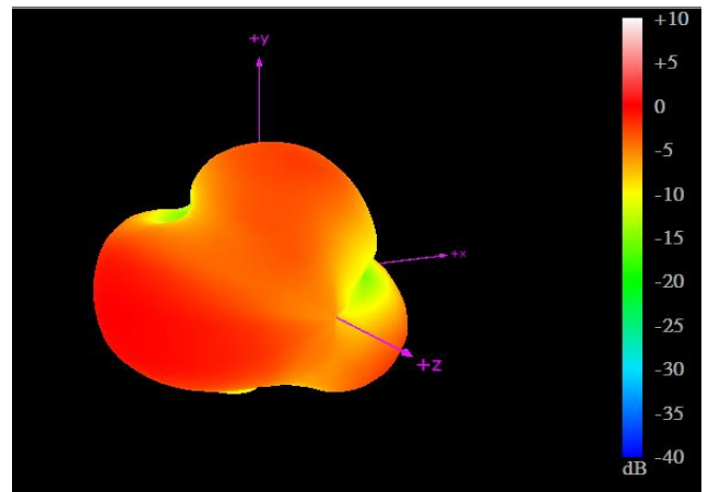
960MHz
