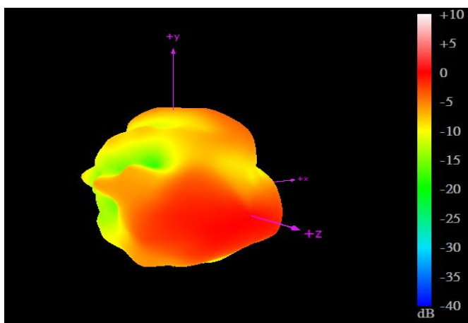
2690MHz
