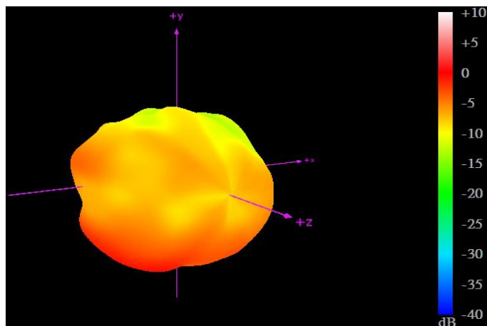
2690MHz
